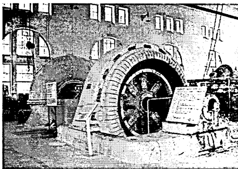
〈発電機室〉
